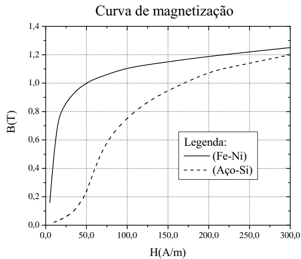
Figura 1: Curvas de magnetização para dois tipos de materiais.
