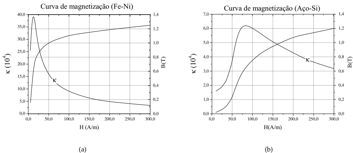
Figura 2: Curvas de magnetização e permeabilidade relativa, para os dois tipos de materiais.
